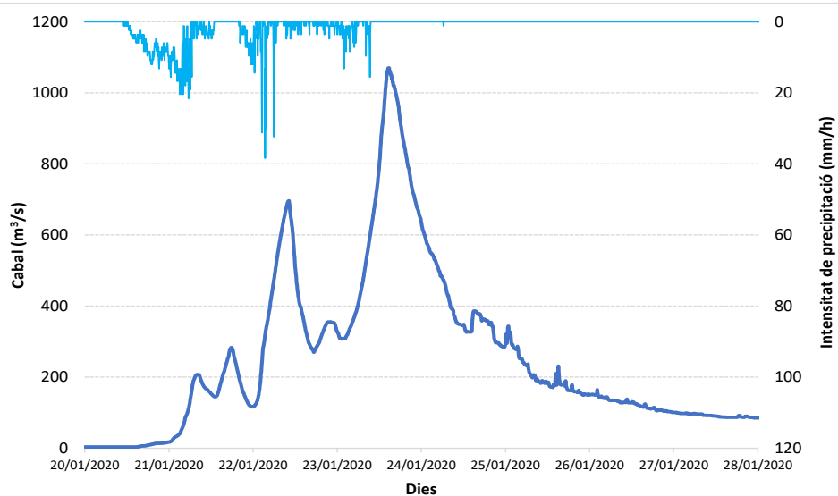
Fig. 9. Hidrograma de crecuda i hietograma del riu Ter a Girona
