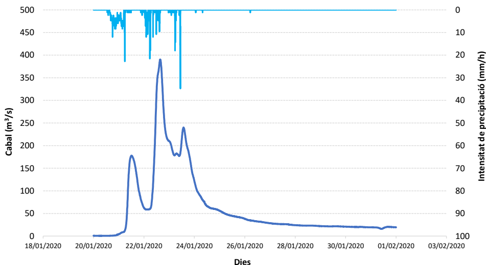
Fig. 12. Hidrograma i hietograma de crecuda de la Muga a Castell d'Empúries
