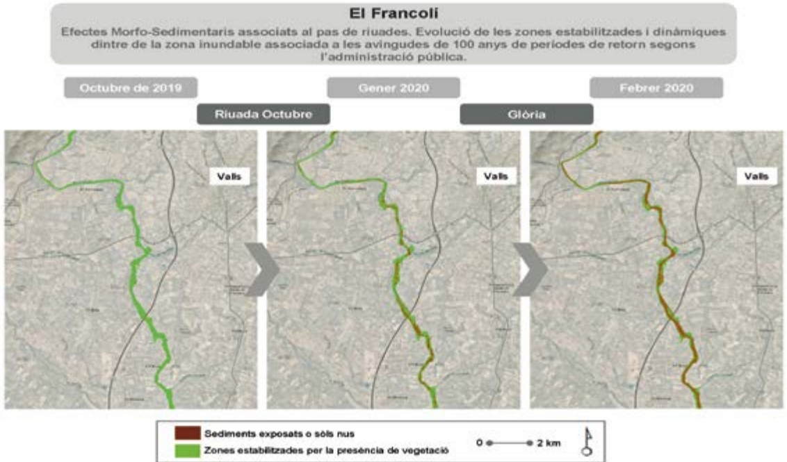
Figura 14. Efectes morfosedimentaris del Glòria al riu Francolí: processos erosius i de sedimentació que afavoreixen l'aparició d'unitat morfològiques i la reconexió transversal de les lleres.
